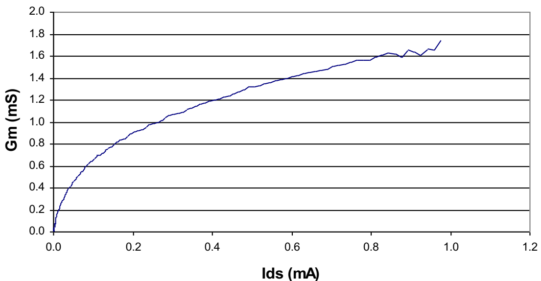
G_m vs I_{ds} , V_{ds}=10V I_{dss}=1mA
