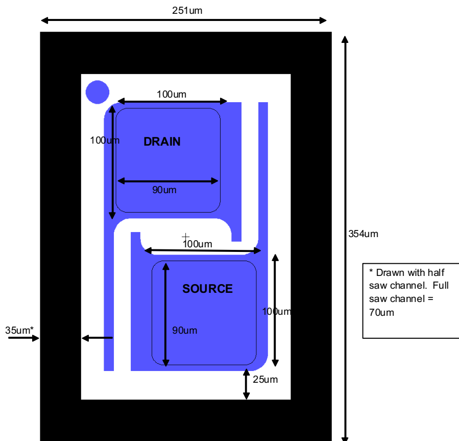
564106 – SHRINK JFET DIMENSIONS
